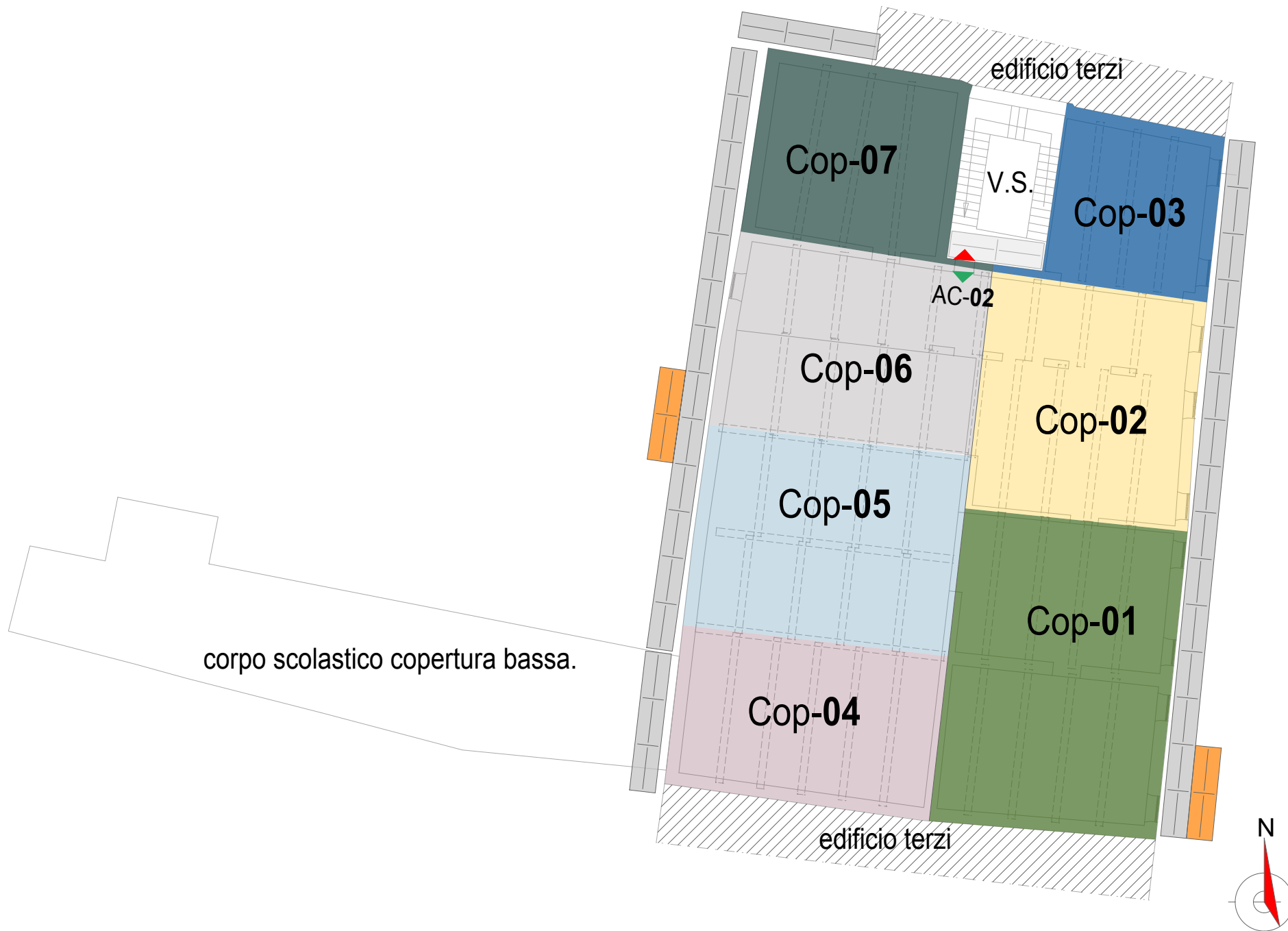
CANTIERE V. Da Feltre - LAYOUT - Piano cop._ripartizione interventi
